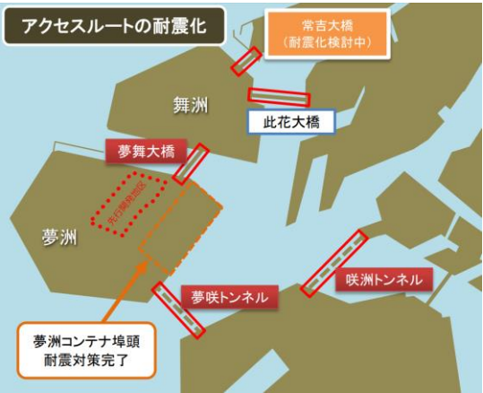
夢洲大橋は平成13年 夢洲トンネルは21年に竣工
