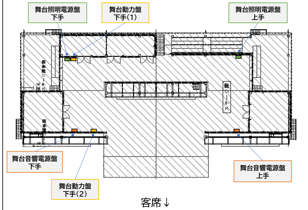
ステージ仮設電源配置図
